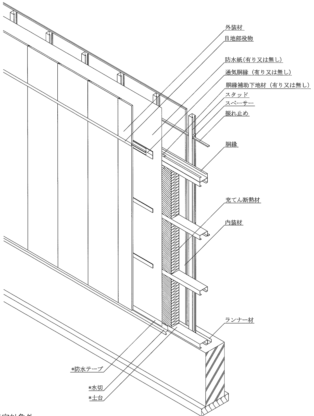
透視図
