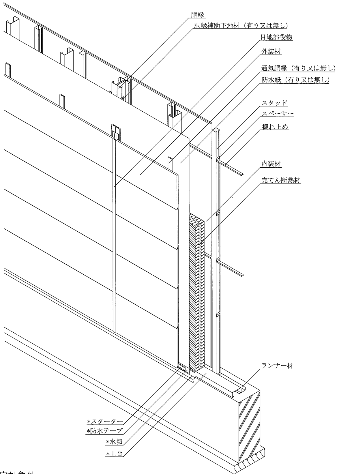
透視図
