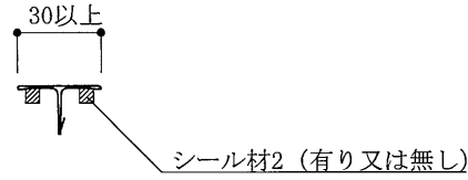
断面図
